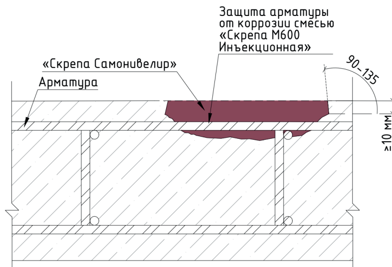
Рисунок А.1.4.2 – Схема восстановления дефектов на горизонтальной поверхности
