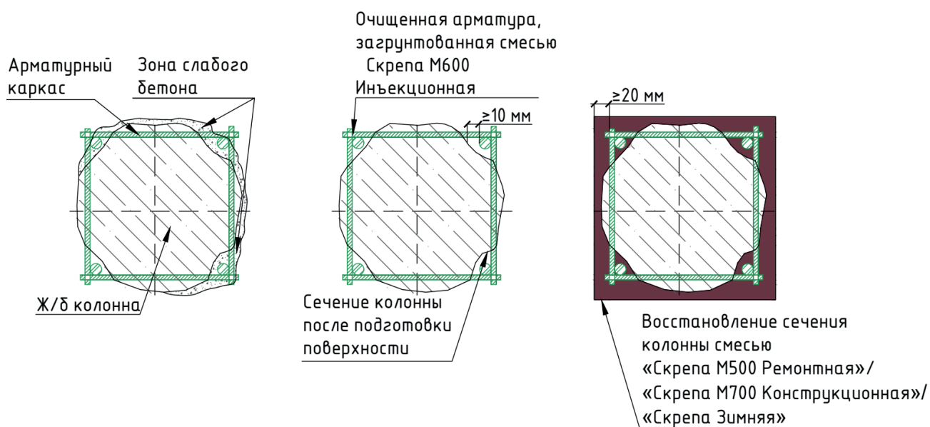
Рисунок А.1.2.3 – Схема восстановления железобетонных колонн
