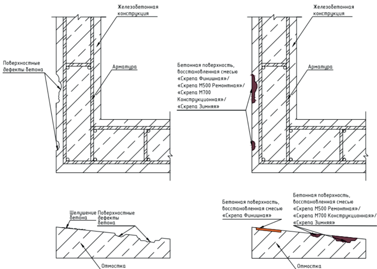
Рисунок А.1.1.1 – Схема устранения поверхностных дефектов бетона поверхностно-восстановительными смесями (шелушение, каверны, раковины и сколы)
