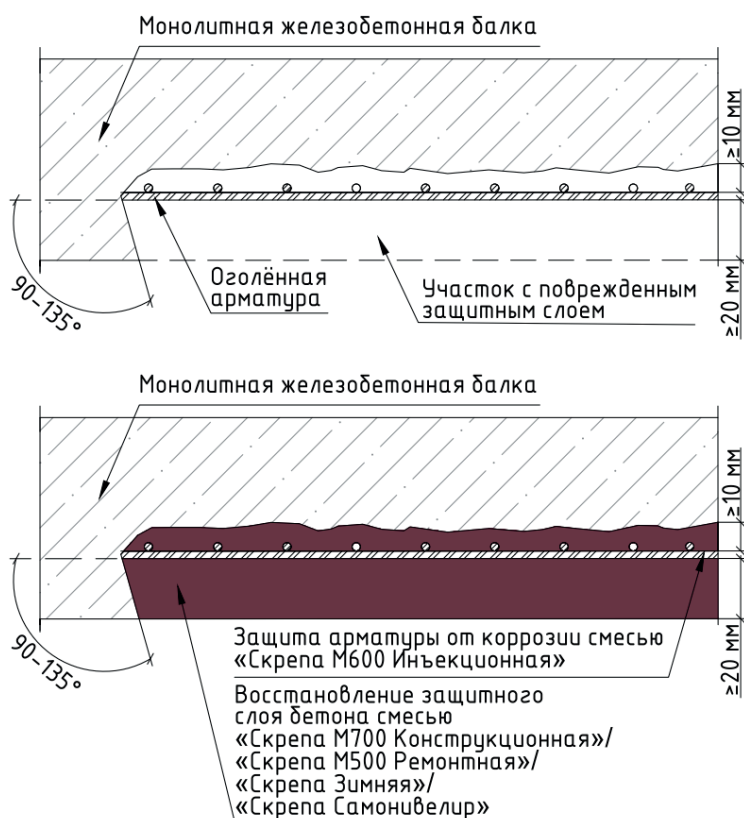
Рисунок А.1.3.2 – Схема восстановления растянутой зоны балки
