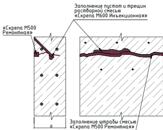
в) Фрагмент бетонной стены после ремонта
