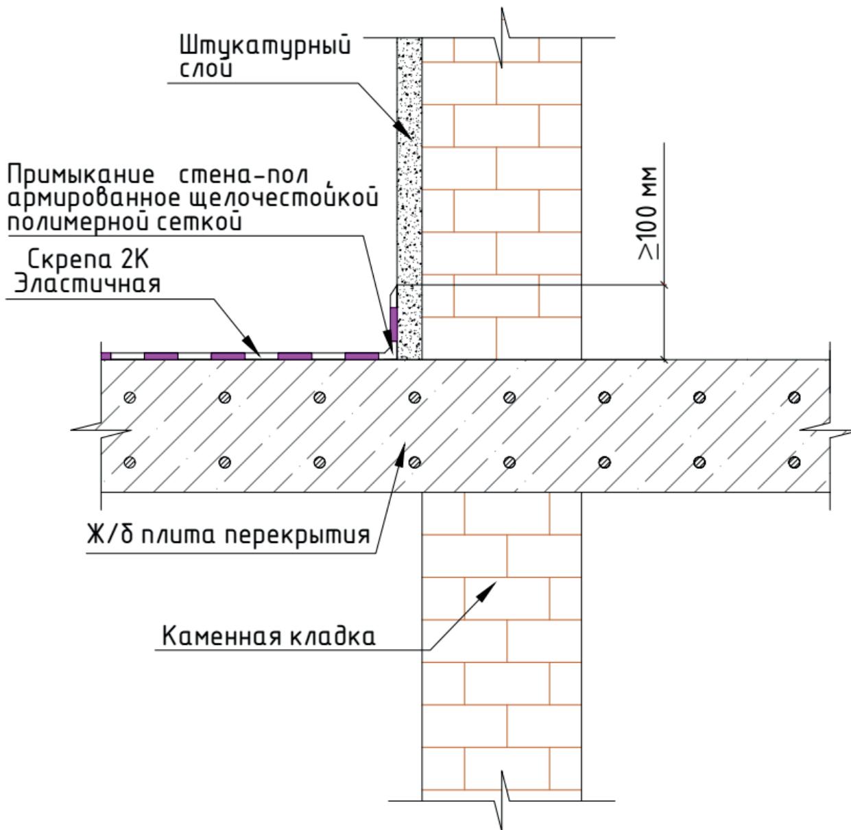
Рисунок А.3.1 – Схема гидроизоляции санитарно-технических узлов
