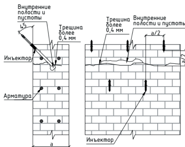
б) фрагмент каменной стены до ремонта, схема монтажа иньекторов
