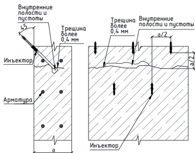
а) Фрагмент бетонной стены до ремонта, схема монтажа иньекторов
