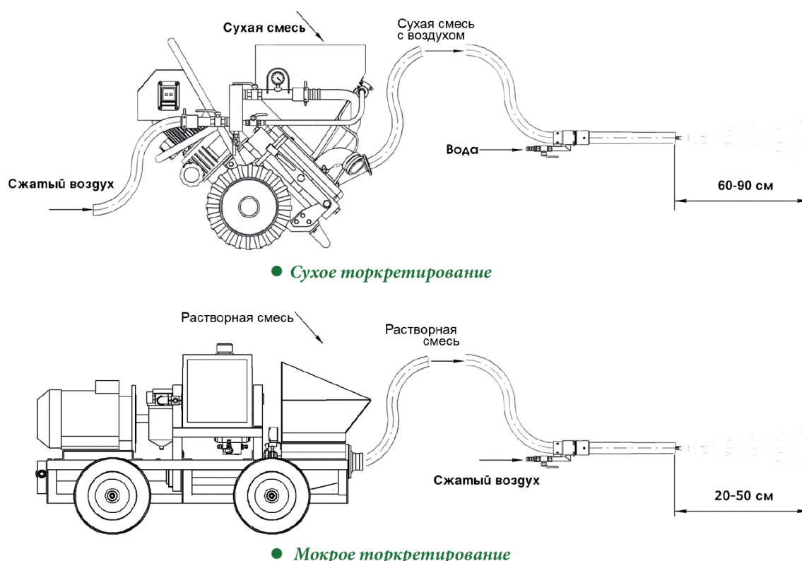
Рисунок В.3 – Технологическая схема сухого и мокрого торкретирования
