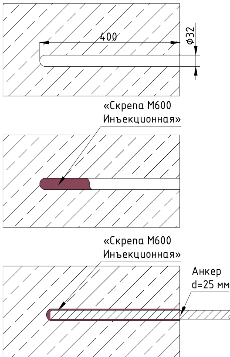
Рисунок А.4 – Схема закрепления анкера в строительной конструкции Технология закрепления анкеров – см. таблицу А.4
