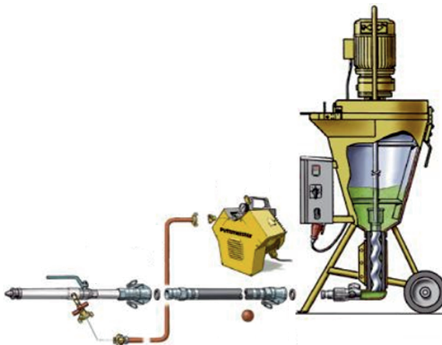
Рисунок В.4 – Технологическая схема штукатурной станции
