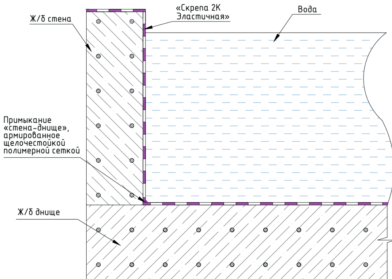
Рисунок А.3.2 – Гидроизоляция наземных монолитных ж/б ёмкостных сооружений
