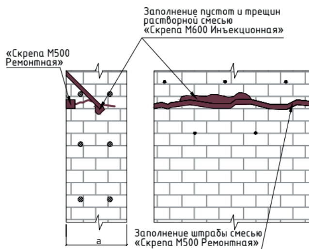
г) Фрагмент каменной стены после ремонта
