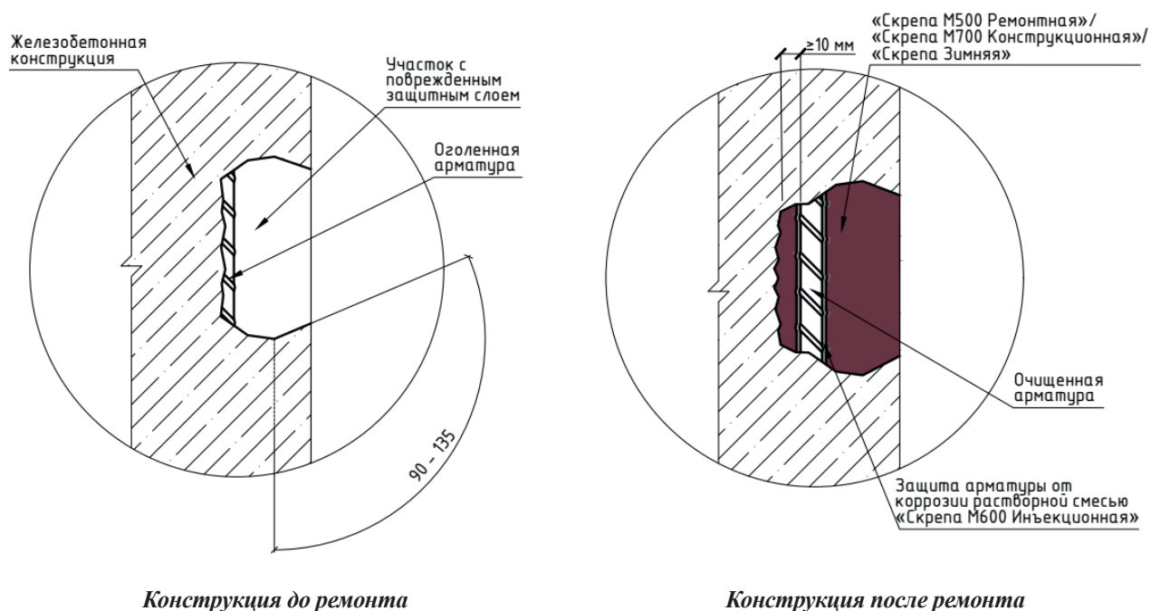
Рисунок А.1.2.2 – Схема восстановления защитного слоя железобетона
