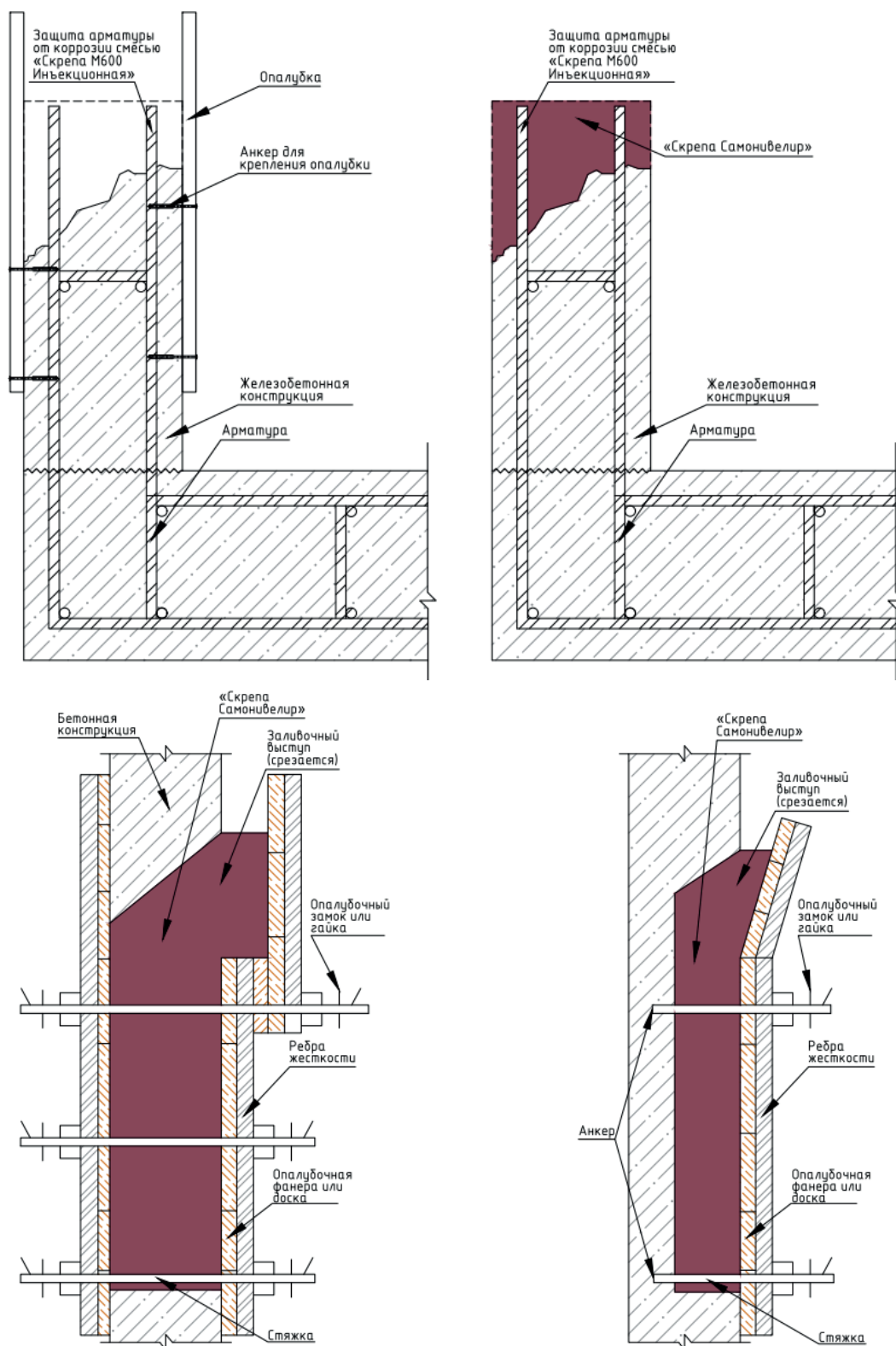
Рисунок А.1.4.1 – Схемы восстановления частично разрушенного бетона вертикальной конструкции
