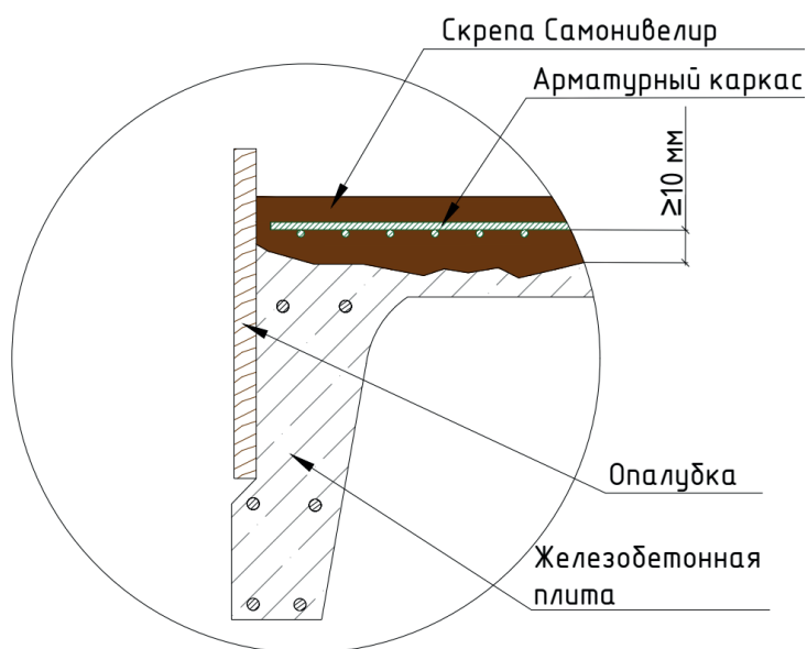
Рисунок А.1.4.4 – Восстановление плиты в сжатой зоне
