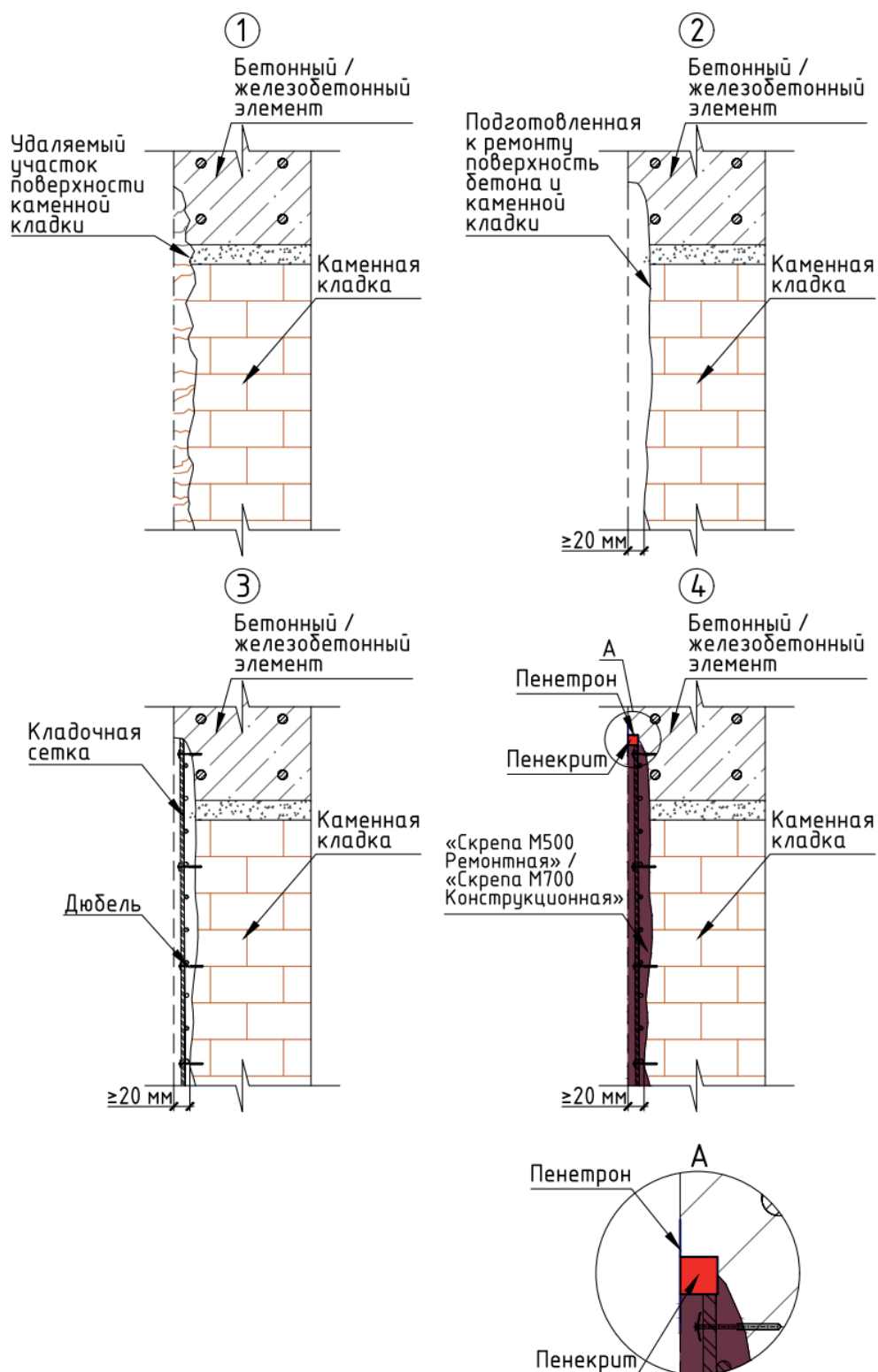
Рисунок А.3.3 – Схема восстановления и гидроизоляции каменной кладки
