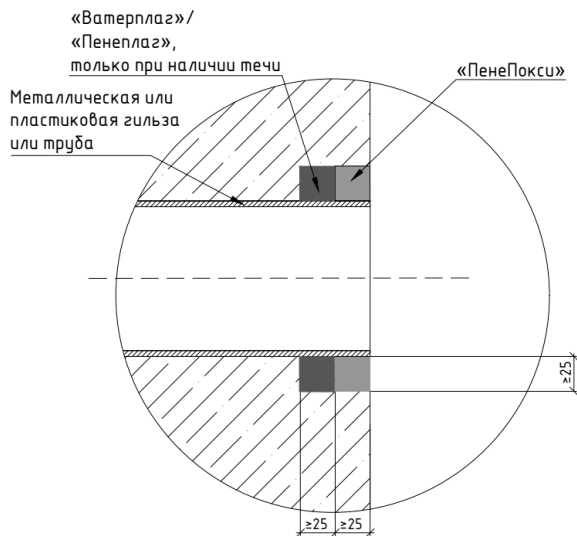
Рисунок 8.8 – Схема гидроизоляции сопряжения металлической/пластиковой гильзы и бетона (вариант 3)
