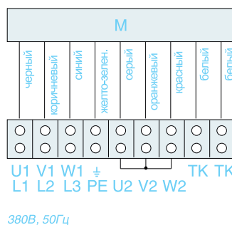
3-фазный двигатель «Звезда»
