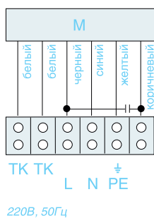
1-фазный двигатель
