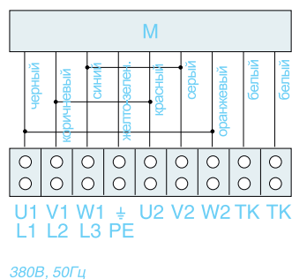
3-фазный двигатель «Треугольник»
