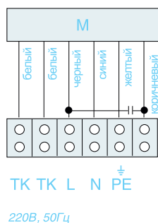
1-фазный двигатель
