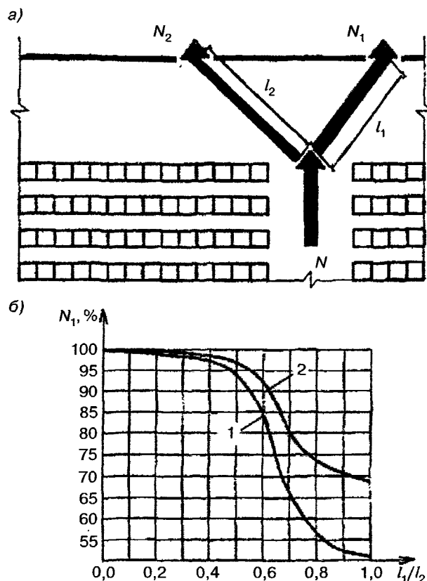
Рисунок Ж.2 — Распределение численности зрителей между выходами
