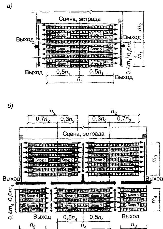
Рисунок Ж.1 — Маршрутизация движения людских потоков при эвакуации из зрительных залов
